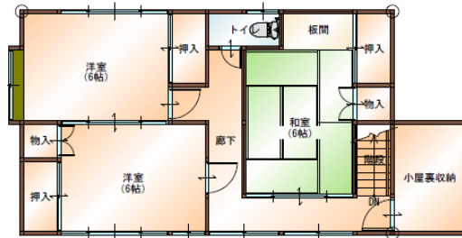
母屋3階
