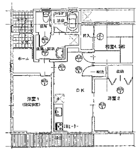
3DK 間取り
