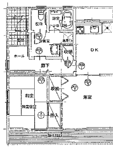
2DK 間取り
