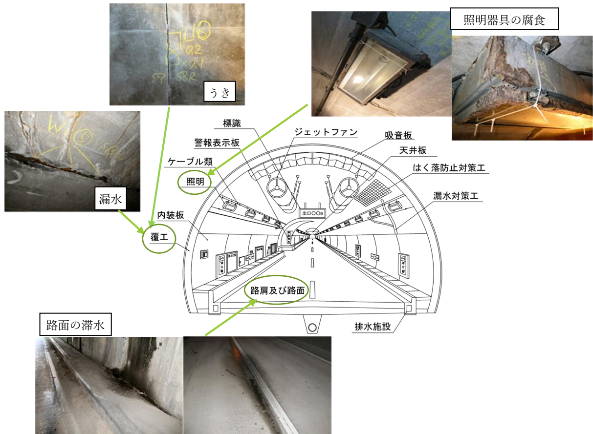
図-1.4 トンネルに発生する変状事例（平成 30 年度藤ヶ峠トンネル点検結果より）
