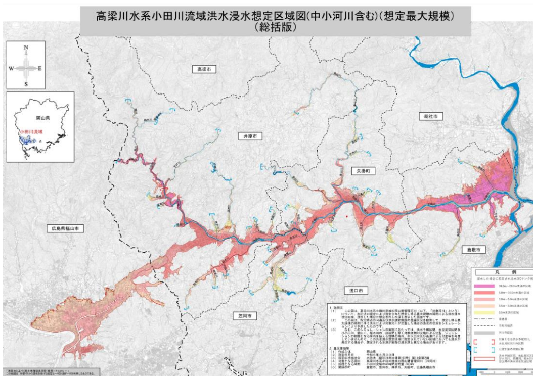
小田川の洪水浸水想定区域（想定最大規模）
