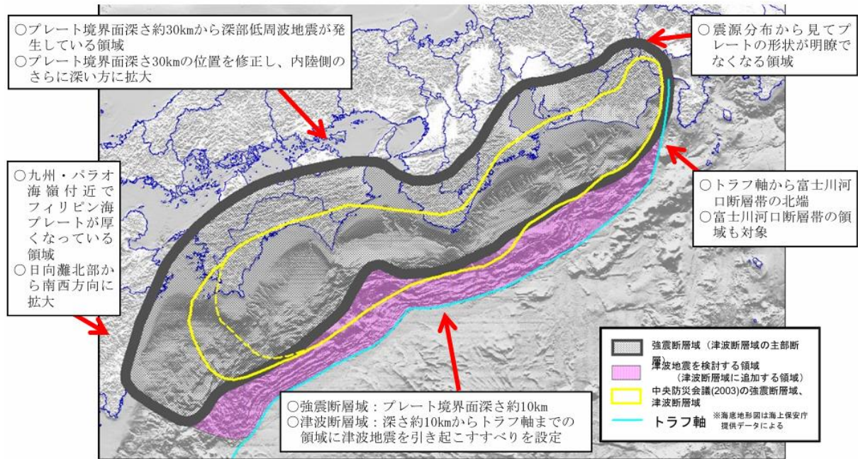
南海トラフ巨大地震の想定震源域
