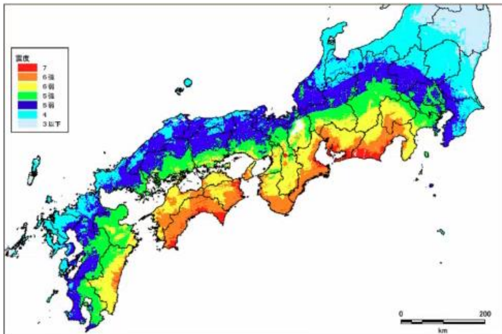
国が想定した「強震波形4ケースと経験的手法の震度の最大値の分布」
